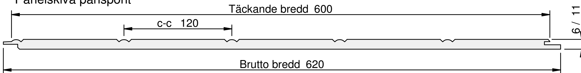
Panelskiva pärlspont
