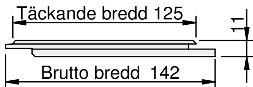
Panelbräda v-fas
