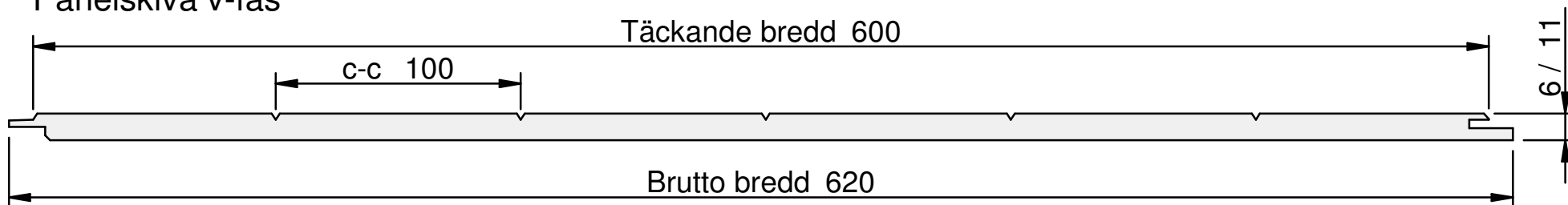
Panelskiva v-fas
