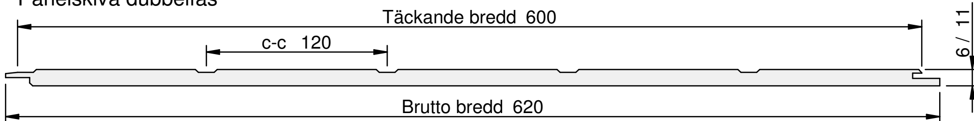
Panelskiva dubbelfas
